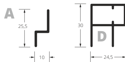
Prowadnice górne.
