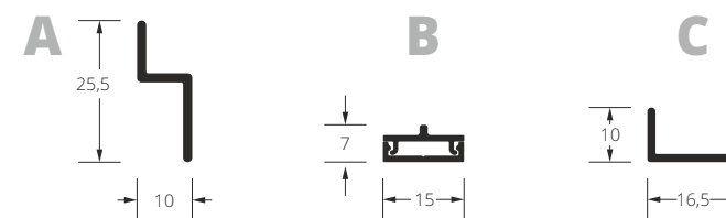
Prowadnice dolne.
