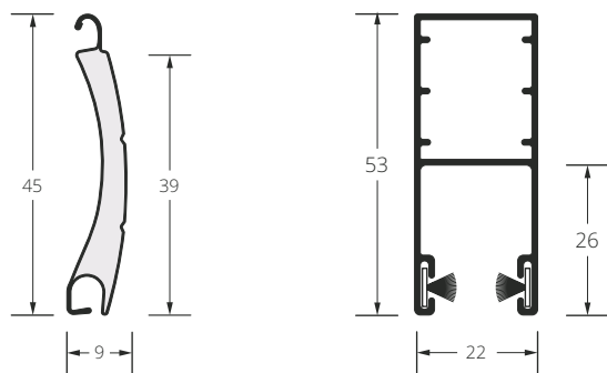
39 mm „PA-39“ aluminum profile.
