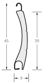
39 mm „PA-39“ aluminum profile.
