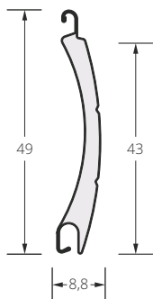
43 mm „PA-43“ aluminum profile.
