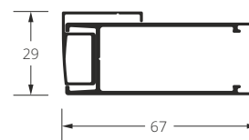
■ guide.
