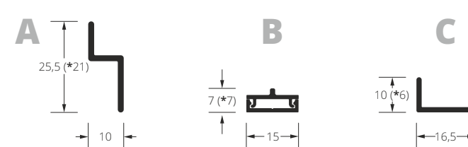
Untere Führungsschienen.
