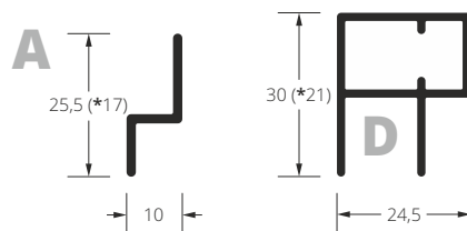
Obere Führungsschienen.
