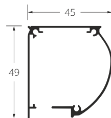
Rys.1 Kasette.
